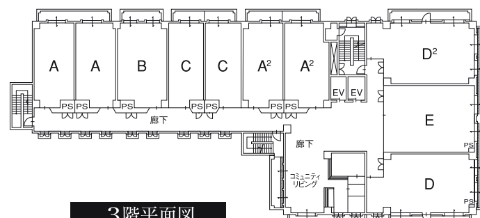
3階平面図
